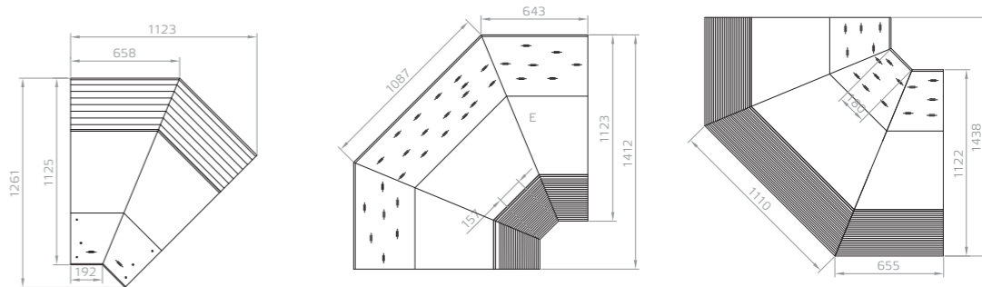
nZITA 45°I nZITA 90°E 3D nZITA 90°I 3D
